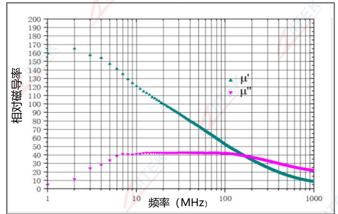
材料磁谱
