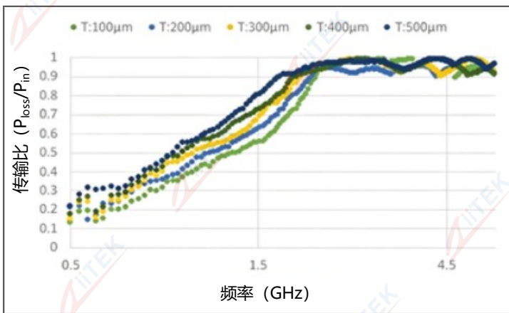
衰减特性
