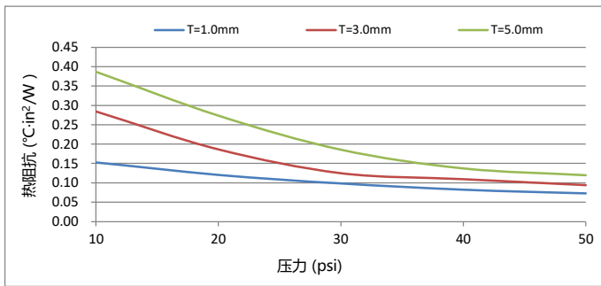
热阻抗
