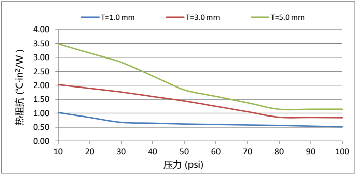
热阻抗
